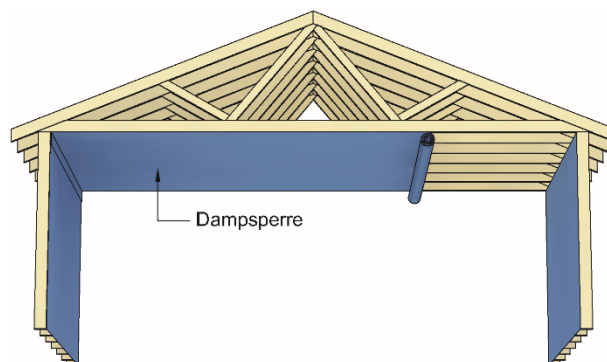
Fig. 1 Kullaplast Dampsperre monterert i yttervegger og mot kaldt loftstrom
