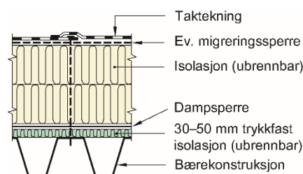
Fig. 2 Kullaplast Dampsperre monterert i kompakt takkonstruksjon
