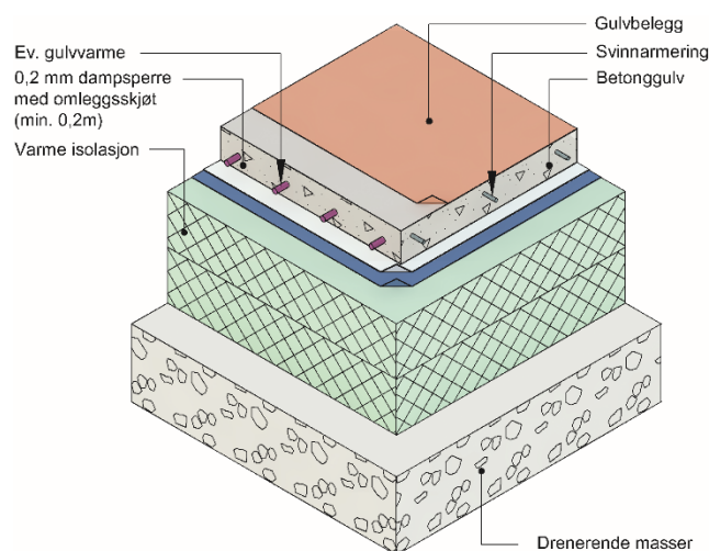
Fig. 3 Kullaplast Dampsperre monterert i betonggulv på grunnen
